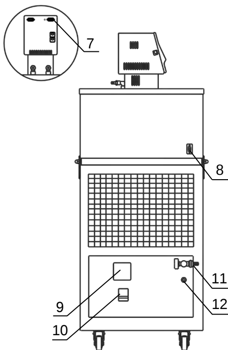
Рисунок 4 — Боковая панель термостата
